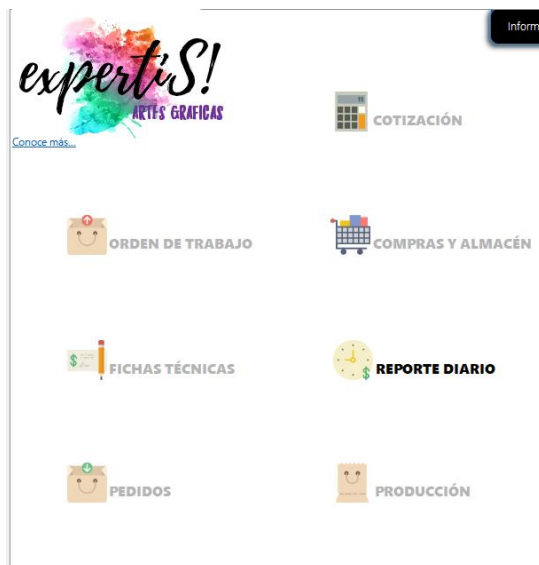
Ilustración 33 Reporte Diario
